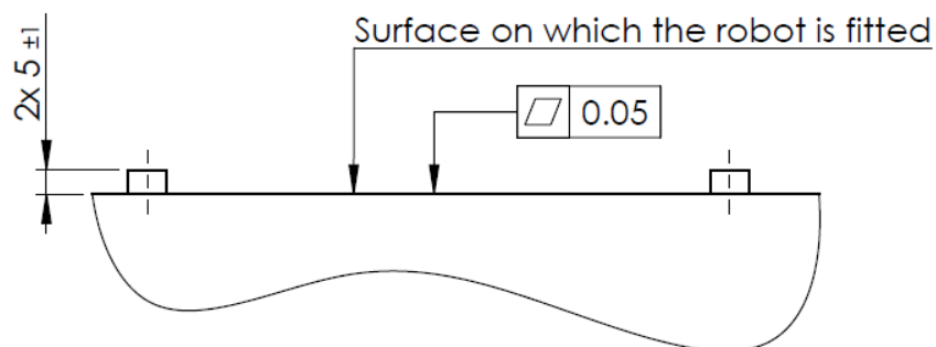
1.2: Monteringsplatta för robotbas
