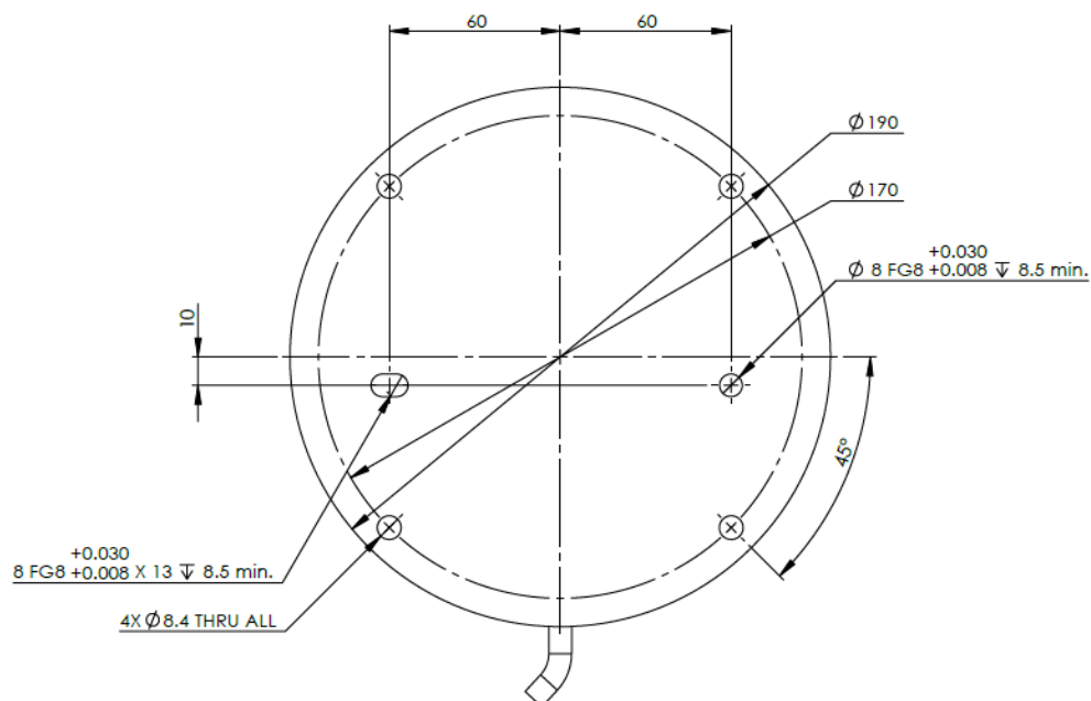
1.1: Undersidan av robotbasen
