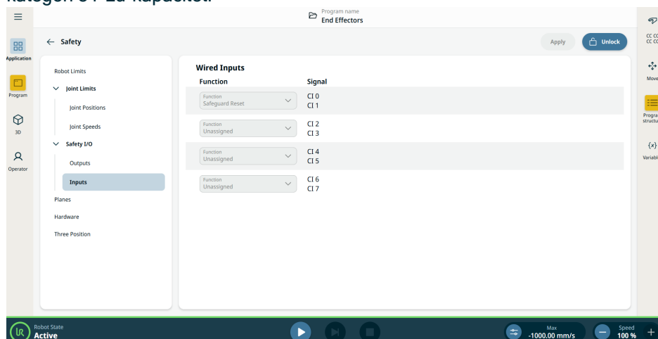
Figur 1.4: PolyScope X-skärm som visar ingångssignaler.
